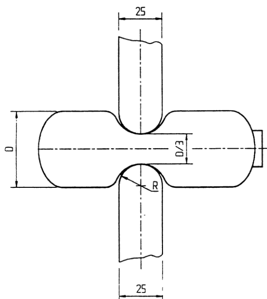
FIGURA 7 – Aplastamiento recipientes cortos
