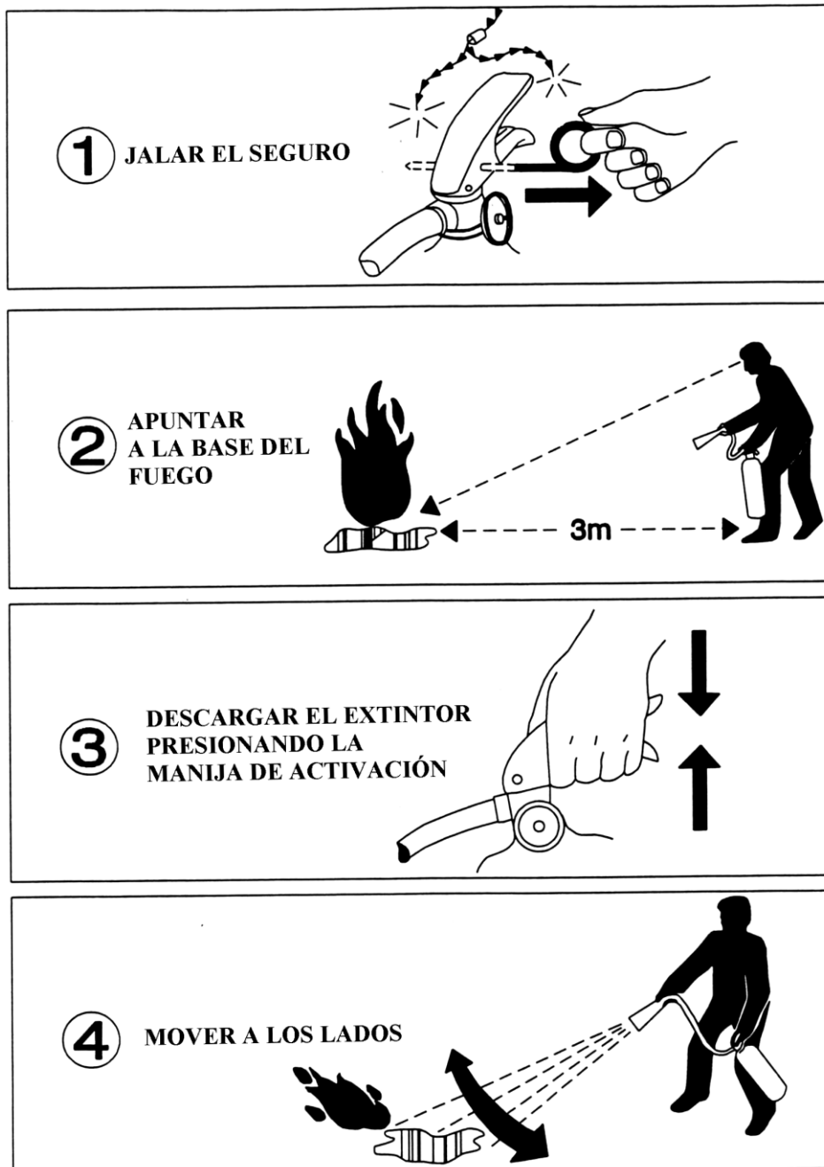
FIGURA 8 – Ejemplo de instrucciones de uso
