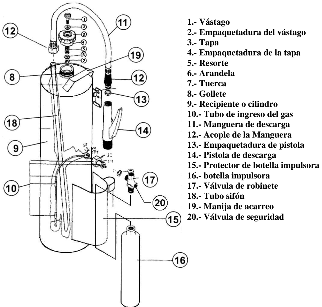
FIGURA 3 – Partes de un extintor portátil manual con botella de impulsión
